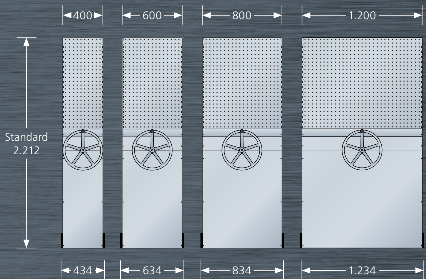
Optionales Schubladensystem zur Lagerung von pharmazeutischen Produkten unter Tiefkühlbedingungen
