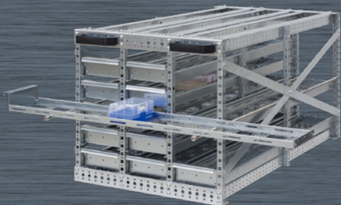
Optionales Schubladensystem zur Lagerung von pharmazeutischen Produkten unter Tiefkühlbedingungen
