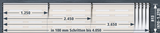
Abmessungen Tablare
